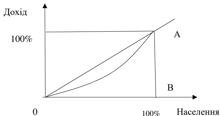
Рис. 2. Крива Лоуренса [6]
